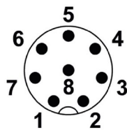
Figura 4.5 Vista del connettore esterno
