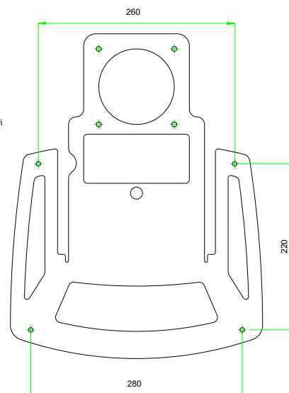
Figura 5.2 Dima foratura
