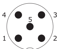
Figura 4.4 Vista del connettore esterno
